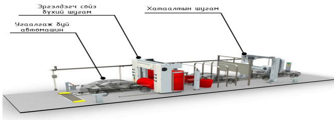
Зураг 4. Автомашиныг механикжсан аргаар угаах үйл ажиллагаа (Жишээ зураг)
