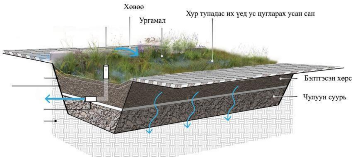
Зураг 22. Үерээс хамгаалах байгууламжийн жишээ зураг
