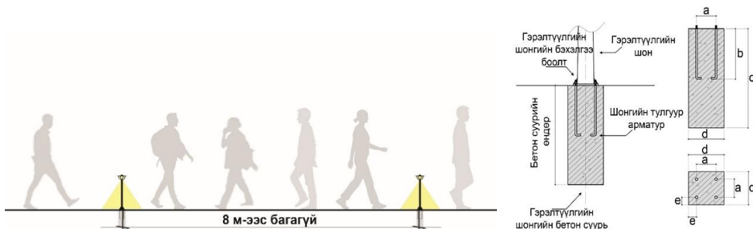
Зураг 9. Гэрэлтүүлэг хоорондын зай болон гэрлийг суурилуулах
