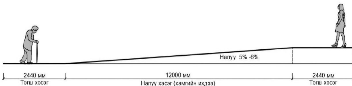
Зураг 8. Дагуу налуу, хөндлөн хэвгий (Жишээ зураг)
