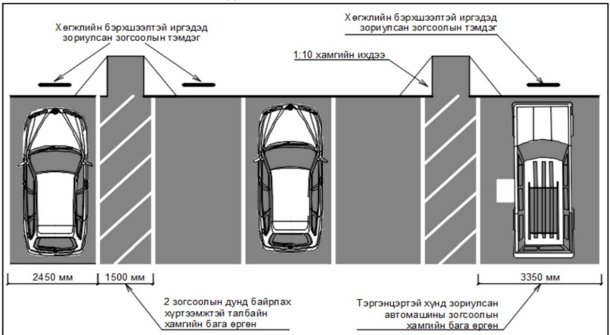
Зураг 3. Хүртээмжтэй зогсоолын хэмжээ (Жишээ зураг)
