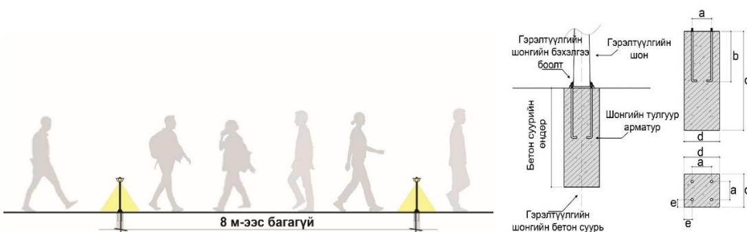
Зураг 9. Гэрэлтүүлэг хоорондын зай болон гэрлийг суурилуулах
