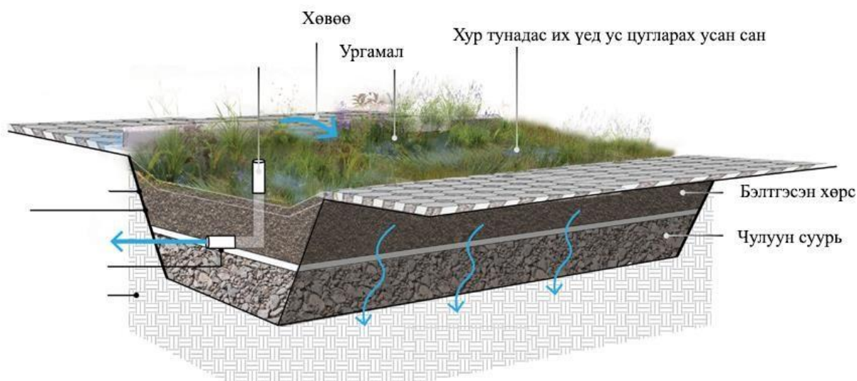
Зураг 20. Үерээс хамгаалах байгууламжийн жишээ зураг
