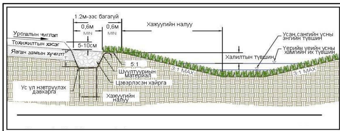
Зураг 6. Борооны ус цуглуулах хөв цөөрмийн тохижилтын огтлолын жишээ зураг
