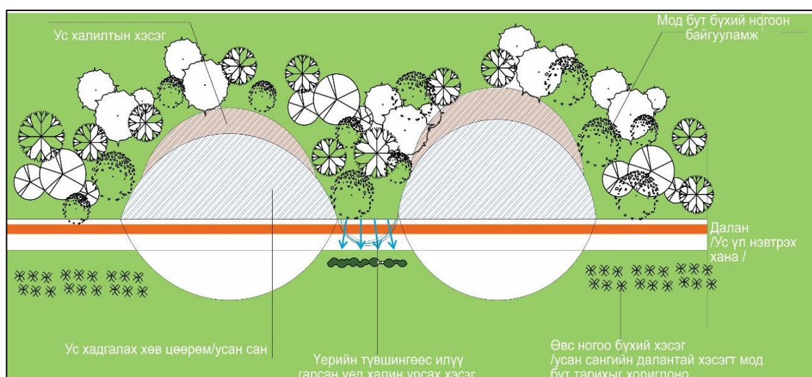
Зураг 11. Суурьшлын бүсийн гадна талбайд ус цуглуулах цөөрөм төлөвлөх жишээ зураг
