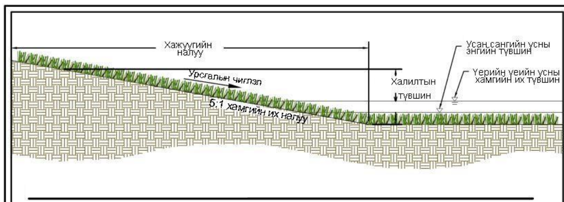
Зураг 7. Борооны ус цуглуулах хөв цөөрөм /жишээ/
