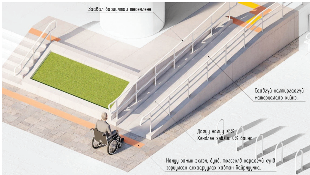
Зураг 6. Барилгын орц, гадна довжоо, налуу замын стандарт (Жишээ зураг)
