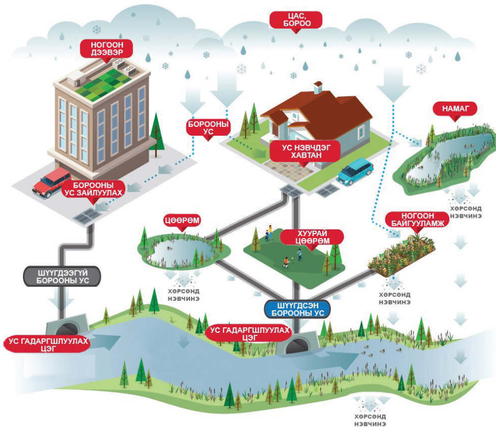
Зураг 4. Үерээс хамгаалах борооны ус зайлуулах байгууламжийн төлөвлөлт (Жишээ зураг)
