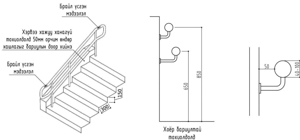
Зураг 5. Шат болон бариулын хэмжээ (Жишээ зураг)
