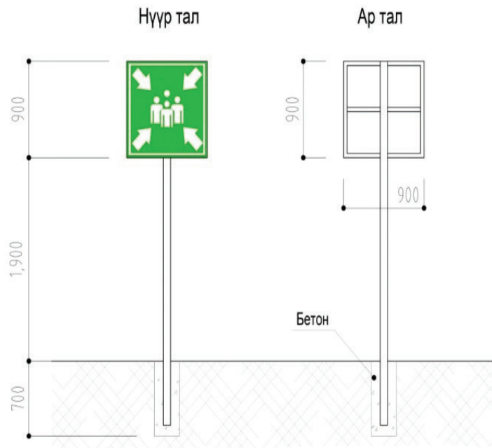
Зураг 27. Түр цугларах аюулгүй талбайн тэмдэг, түүний суурилуулалт (Жишээ зураг)
