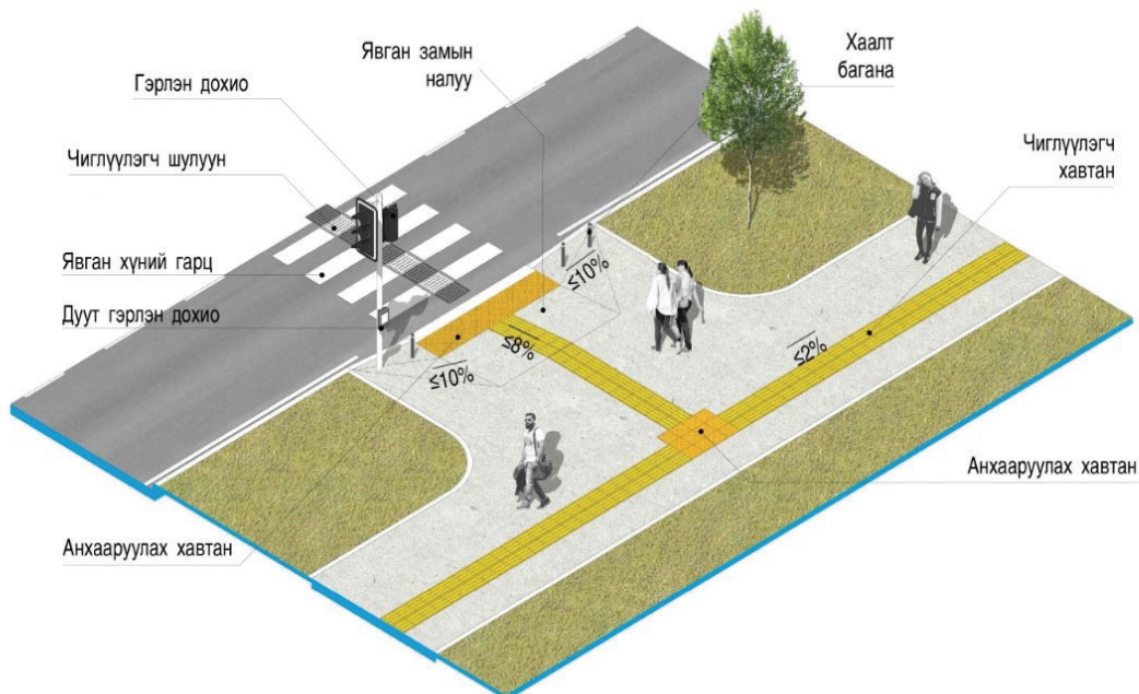
Зураг 9. Явган хүний замын төлөвлөлт, зай хэмжээс (Жишээ зураг)
