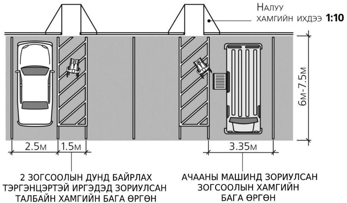
Зураг 14. Хөгжлийн бэрхшээлтэй иргэдэд зориулсан зогсоолын геометр хэмжээ (Жишээ зураг)
