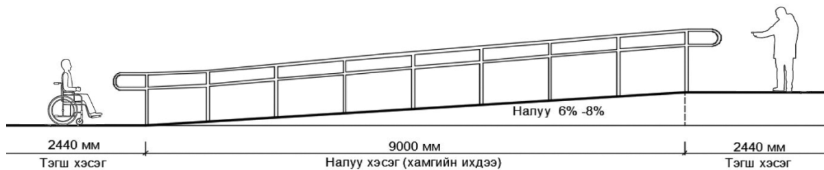
Зураг 7. Шатны нэмэлт бариулын стандарт (Жишээ зураг)
