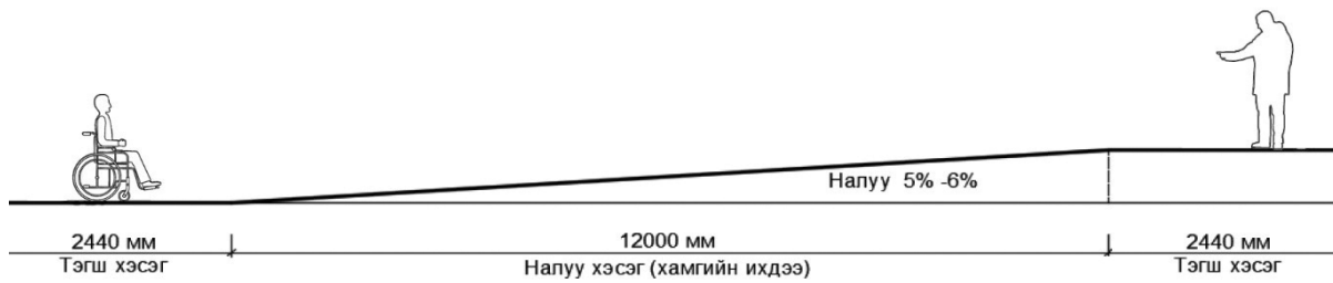
Зураг 8. Налуугийн хэмжээс (Жишээ зураг)
